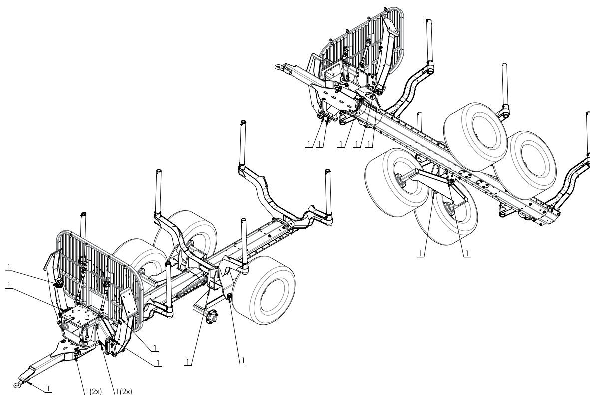
Smörjschema för T10-14 G2.
