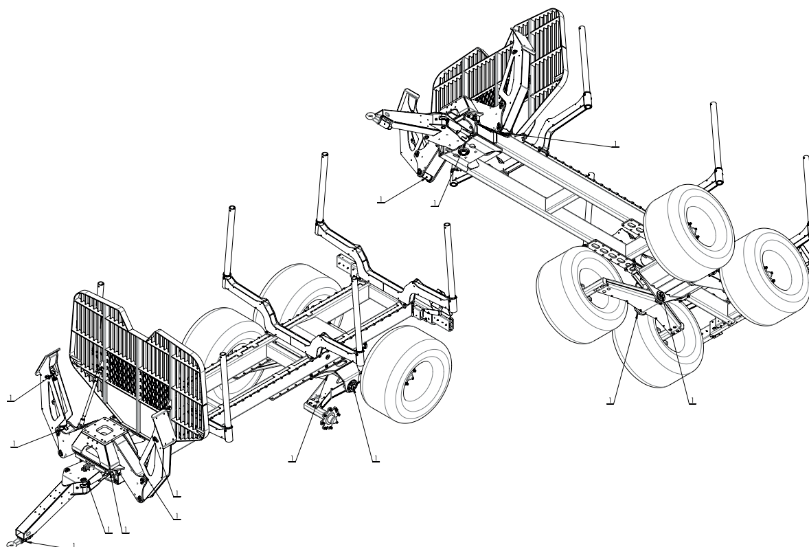
Smörjschema för T17
