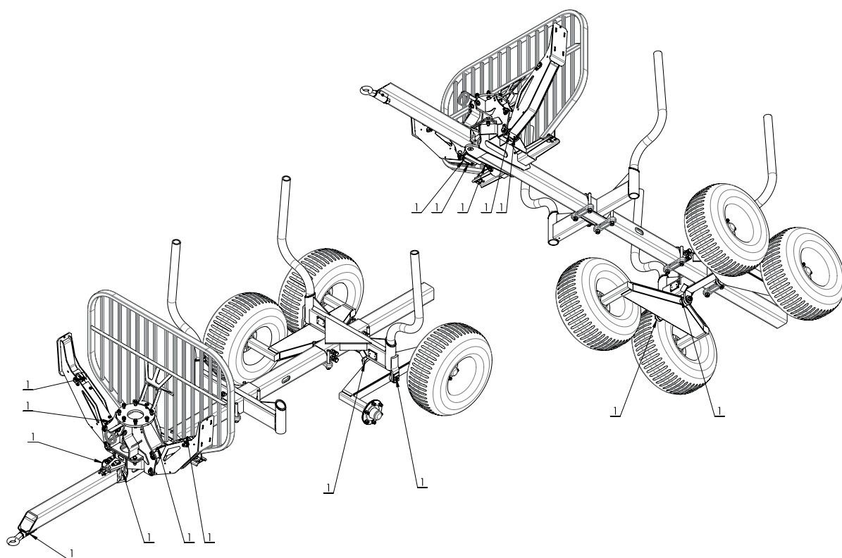
Smörjschema för T7-T8.
