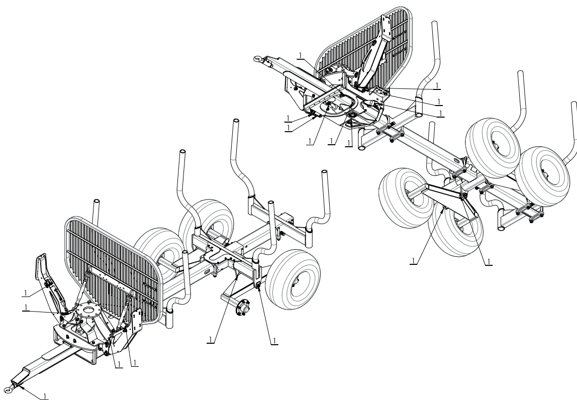
Smörjschema för T9-T10.
